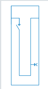
母线联络柜 “L(k)”
